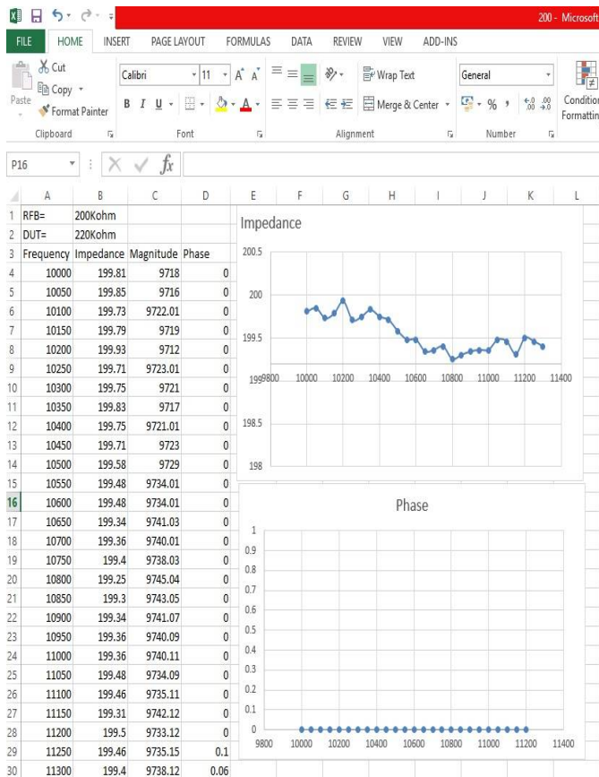
Fig 5 : calibration result
